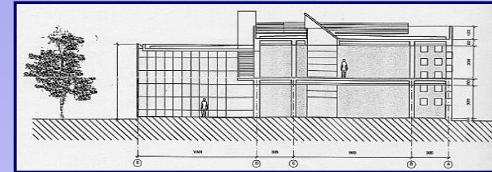
ELEVACION ORIENTE
